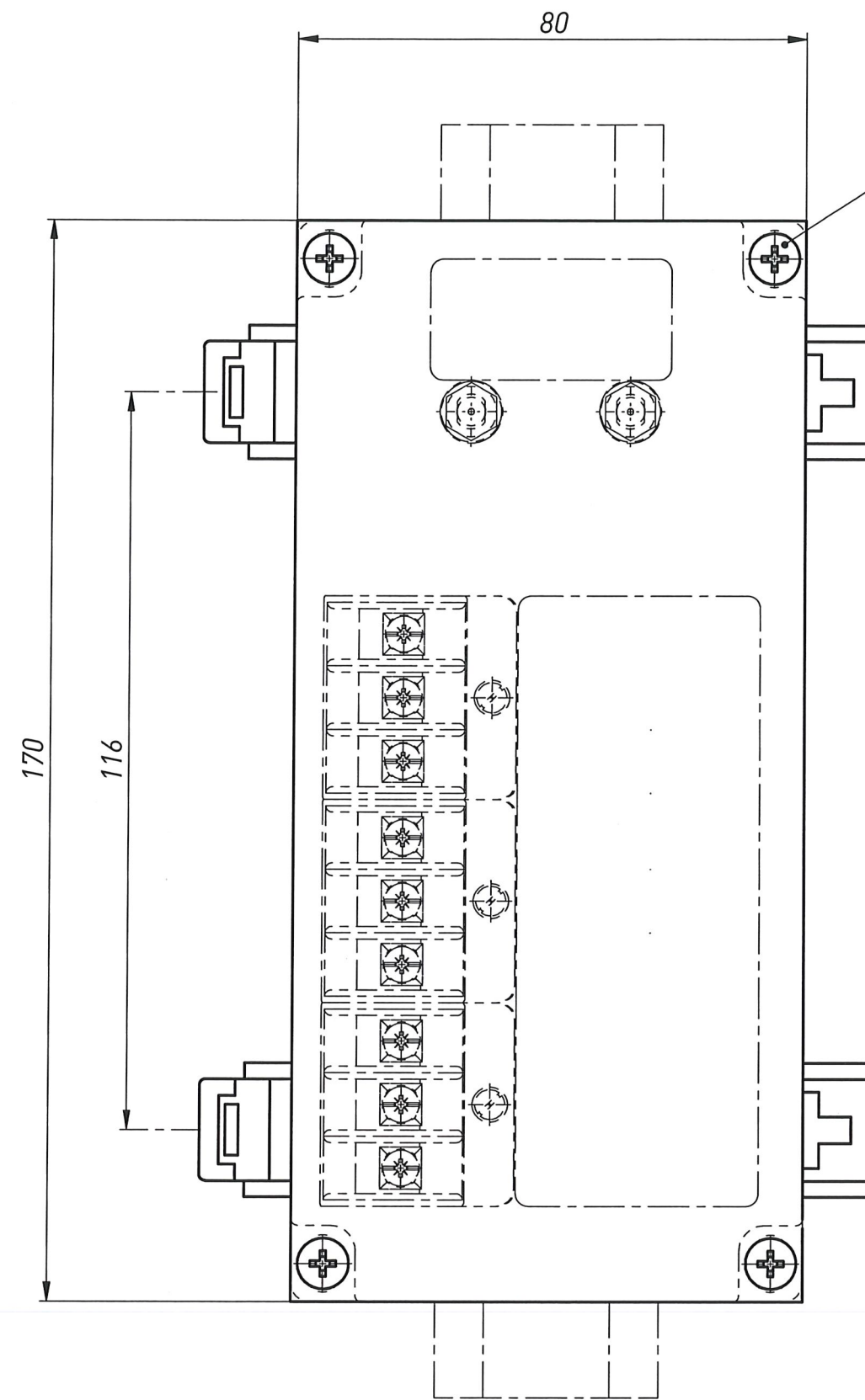
VUE A
